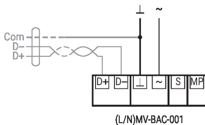
BACnet MS/TP / Modbus RTU
